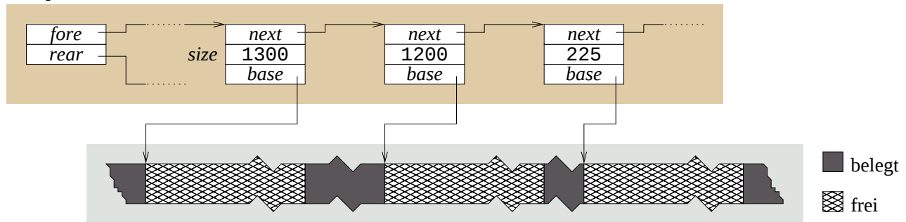
Freispeicherliste
