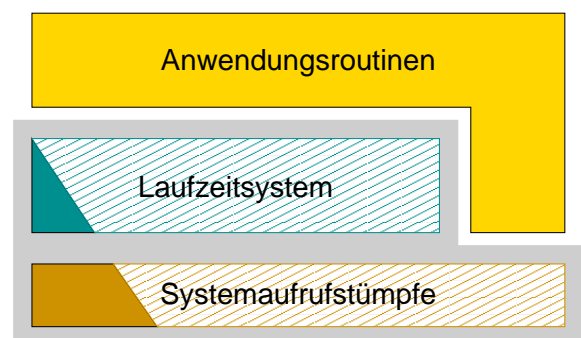
dynamische Bibliothek
