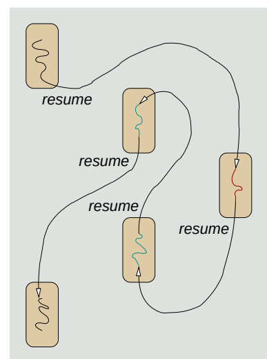
Koroutinen
